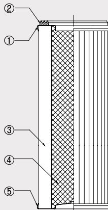
하부 JOINT
